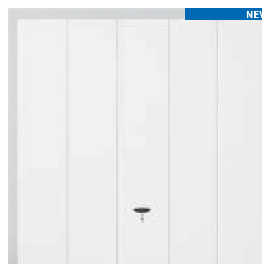
Venus ■ ■
